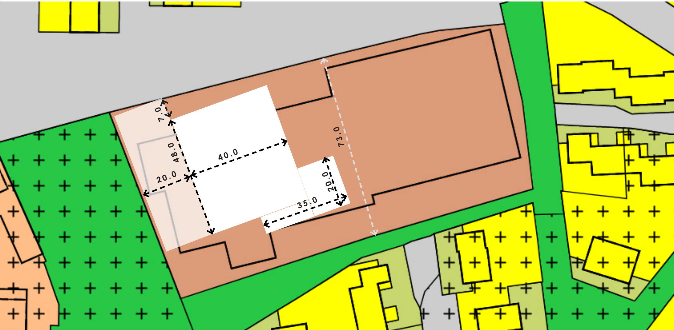
BONGERD afmetingen
