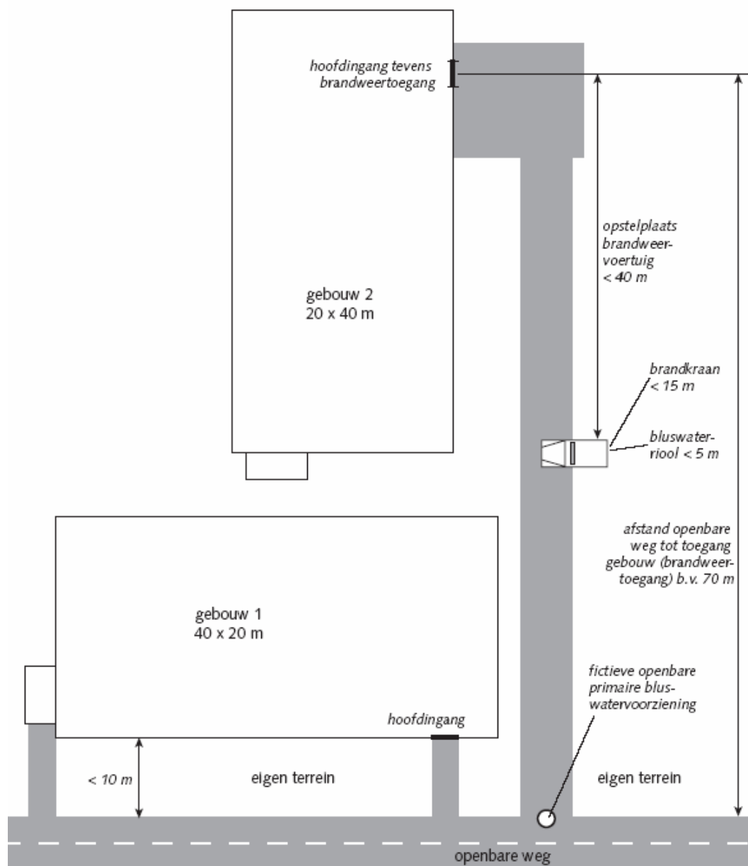
Figuur 2. Projectie niet-openbare bluswatervoorziening
