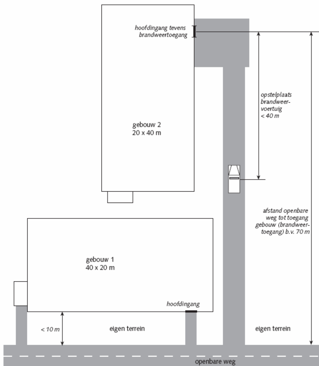
Figuur 1. Projectie opstelplaats eigen terrein
